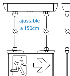
Velos + Cable para suspensión ajustable 150cm (O-ESA-RSA)
